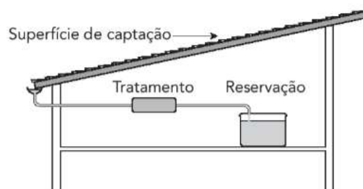
Figura: Esquema com sistema de tratamento e reservatório de armazenamento de água de chuva.
